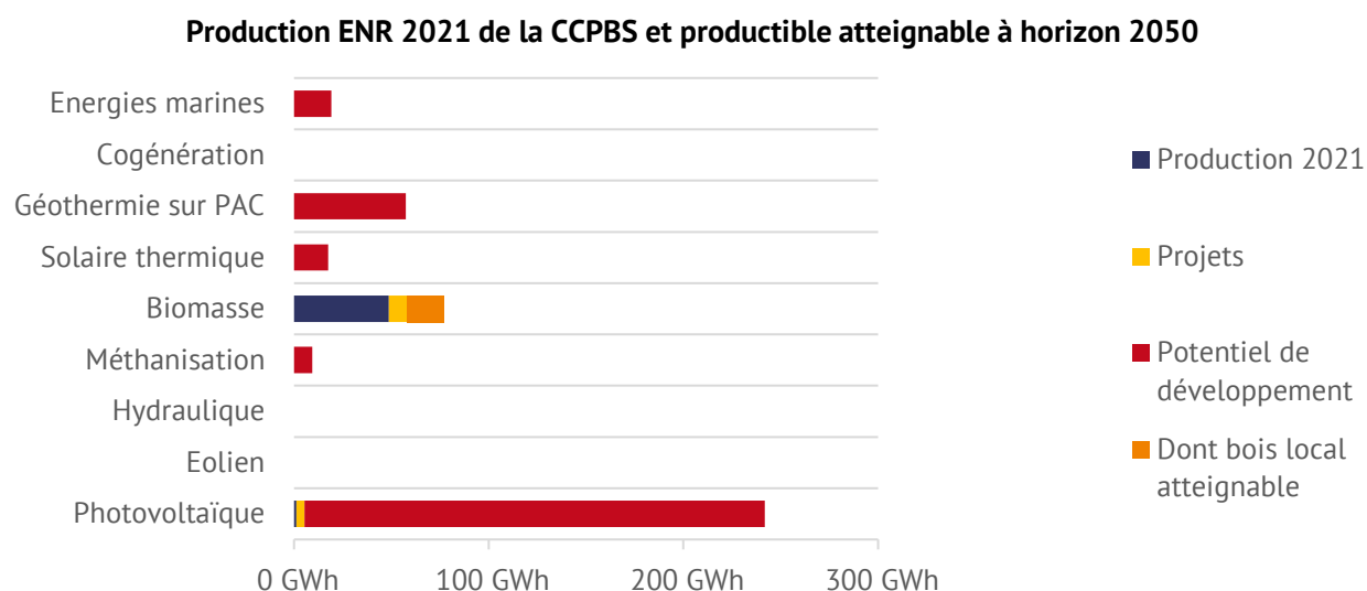
Figure 11 : Synthèse du potentiel de développement des énergies renouvelables, CC Pays Bigouden Sud : NEPSSEN sur la base des données de données multiples
