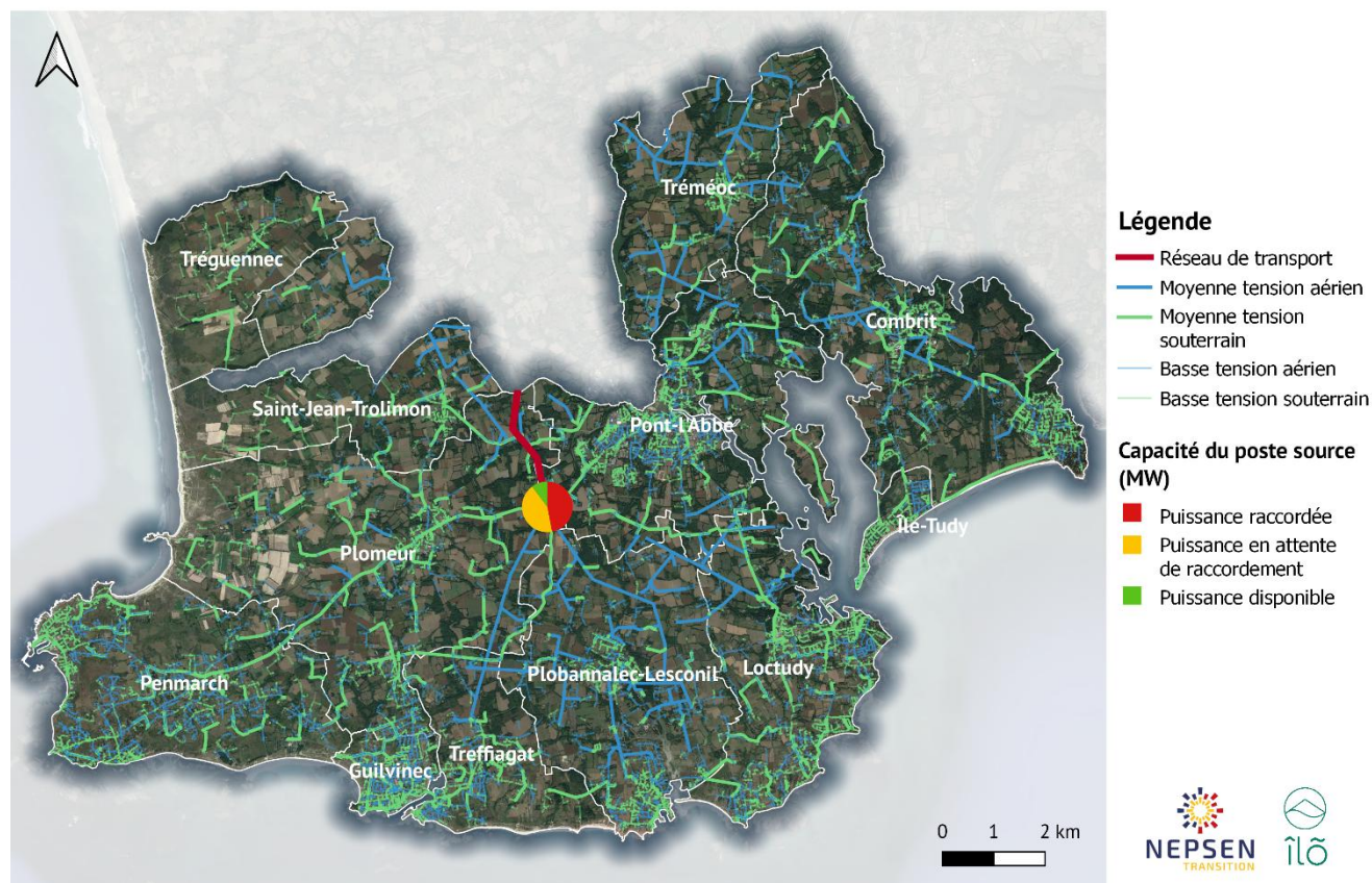
Figure 14 : Synthèses : Capacité de raccordement des postes sources : source : Caparéseau, consulté le 16/01/2023, cartographie NEPSN
