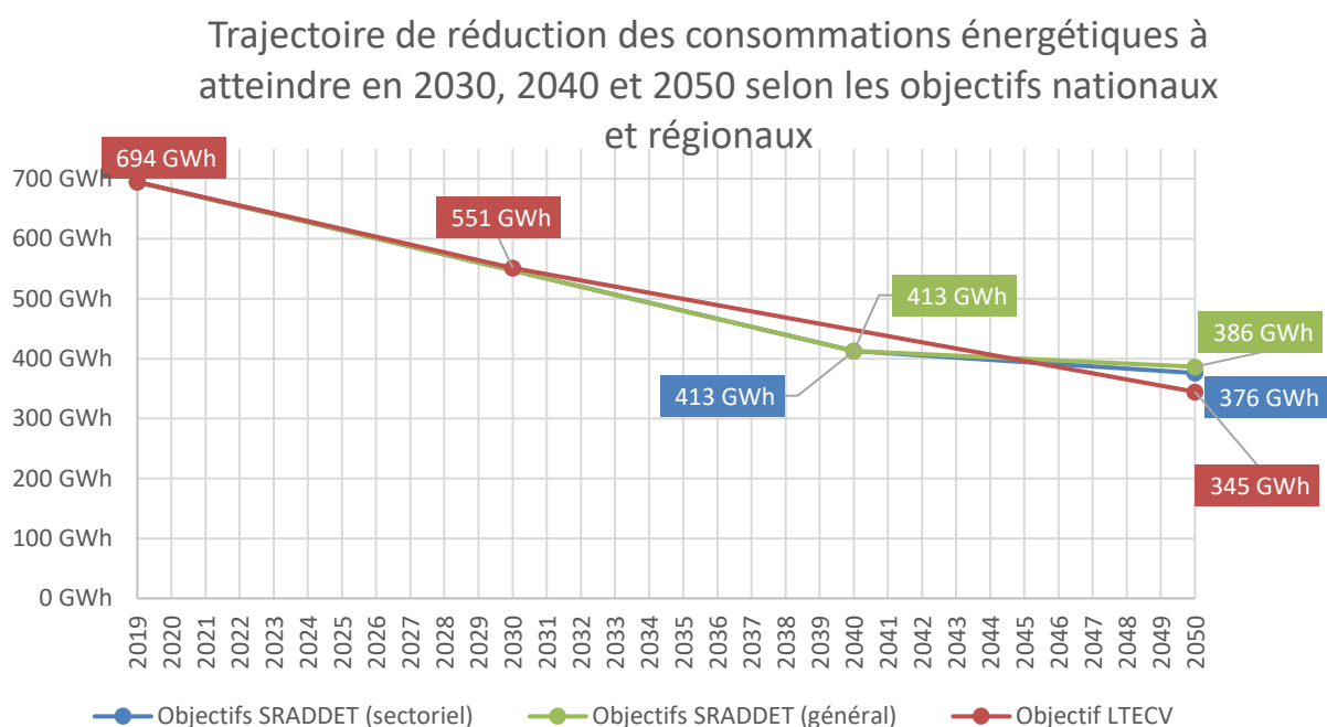
Figure 7 : Trajectoire des consommations d'énergie (en GWh) selon les objectifs régionaux du SRADDET Bretagne et les objectifs nationaux de la LTECV sur le territoire de la communauté de communes du Pays bigouden sud selon l'approche réglementaire
