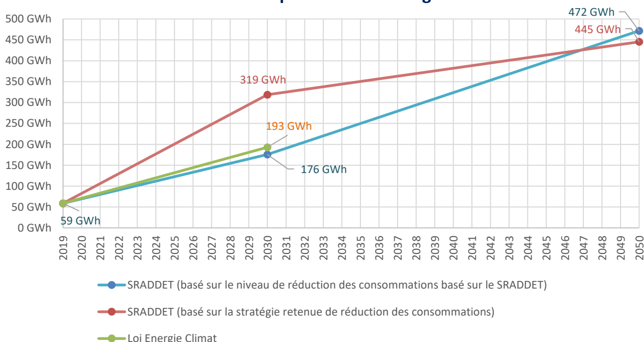
Figure 10 : Trajectoire de la production d'énergie renouvelable (en GWh) selon les objectifs régionaux du SRADDET et les objectifs nationaux de la loi Energie Climat sur le territoire de la Communauté de communes Pays Bigouden Sud
