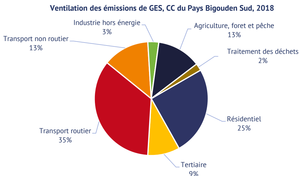
Figure 16: Synthèse – Ventilation des émissions de gaz à effet de serres directes et indirectes associées à l'énergie, Pays bigouden sud, OEB, 2018
